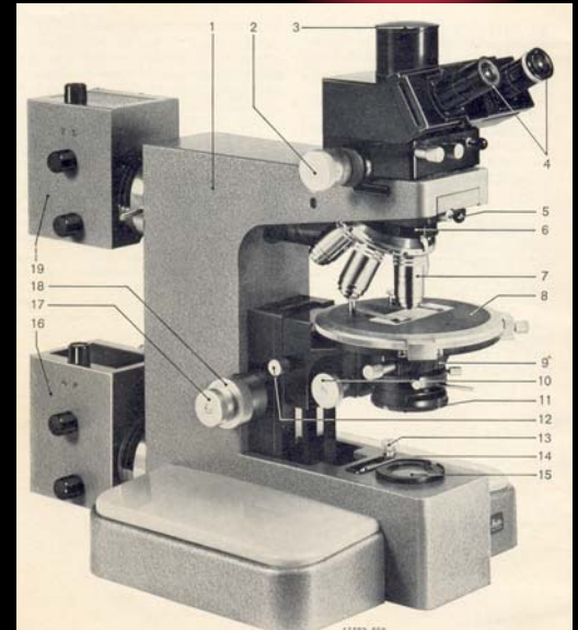
Fig. 1 ORTHOPLAN-POL
